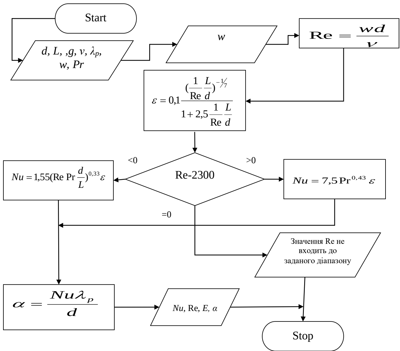
Рис. 4.1. Блок – схема алгоритму до прикладу з використанням арифметичних операторів управління
